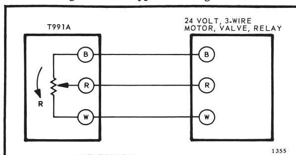
FIG. 9—TYPICAL HOOKUP.
