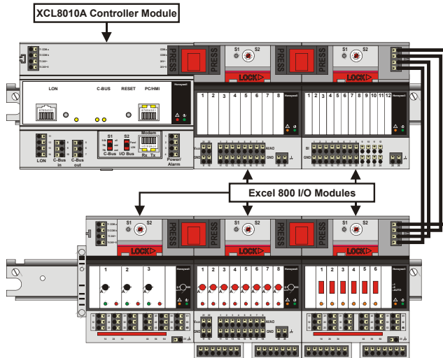
Fig. 8. Excel 800 Controller and I/O Modules on DIN rails
